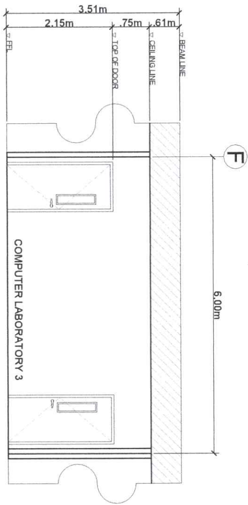
2 SECTION THRU 'X-X' A06 SCALE: 1:70MTS
