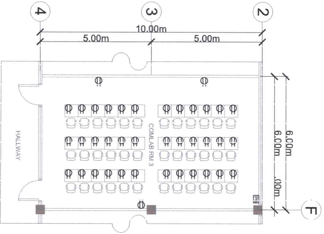
1 EXISTING COMLAB 3 POWER LAY-OUT E03 SCALE: 1:120M/TS
